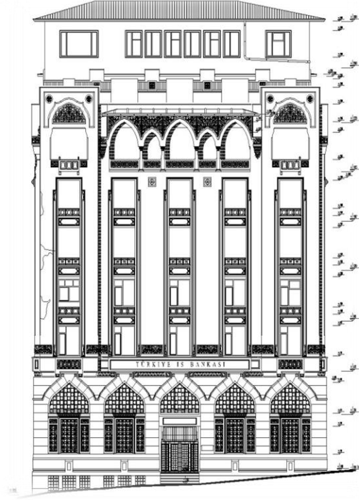
BANKALAR CADDESİ, İŞ BANKASI GALATA ŞUBESİ RÖLÖVESİ
