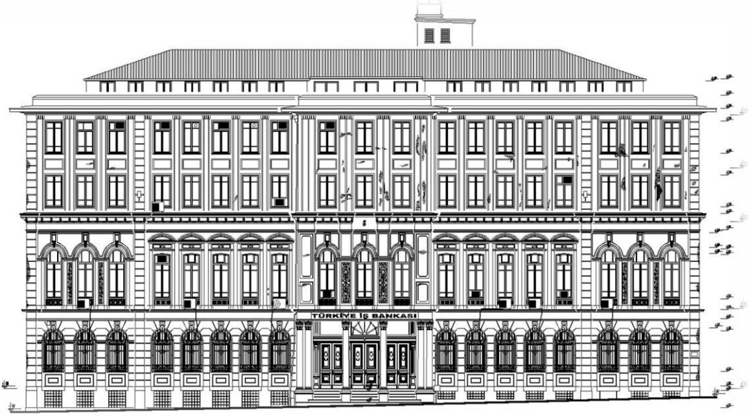
EMİNÖNÜ, İŞ BANKASI YENİ CAMİ ŞUBESİ – RÖLÖVE
