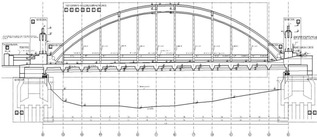
SİLAHTARAĞA FİL KÖPRÜSÜ - RÖLÖVE, RESTİTÜSYON VE RESTORASYON PROJELERİ
